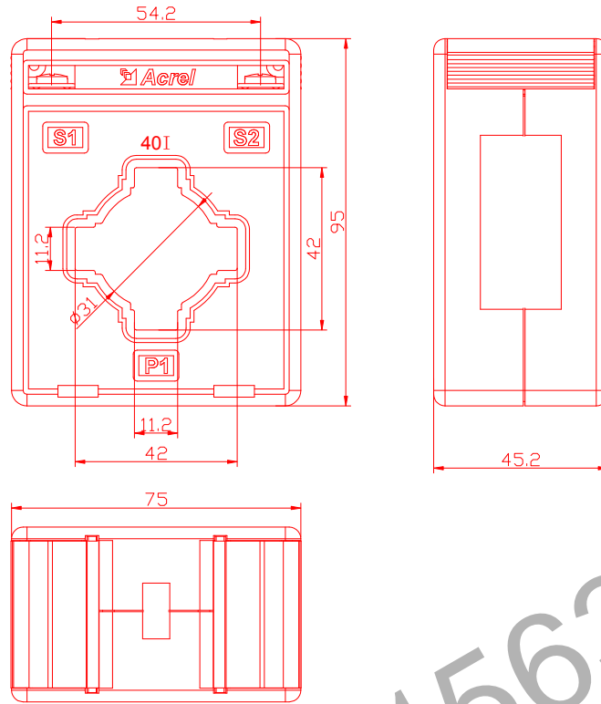
图 6 250A 外置电流互感器外形尺寸
