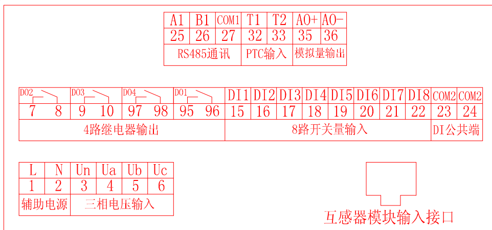
图 3 ARD3 接线端子
