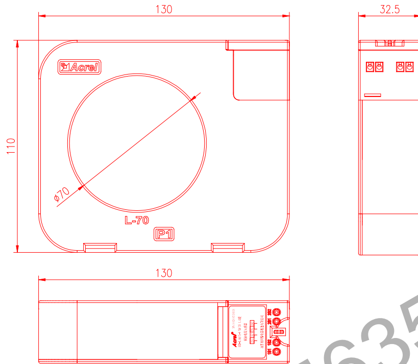
图 8 外置零序电流互感器外形尺寸
