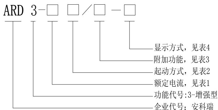
图 2 ARD3 型号说明
